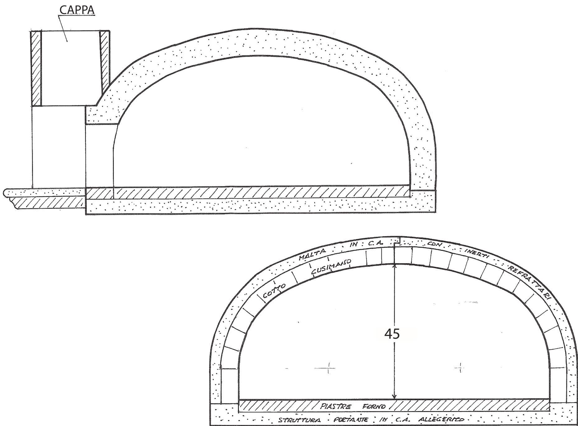
SEZIONE LONGITUDINALE MOD 120
